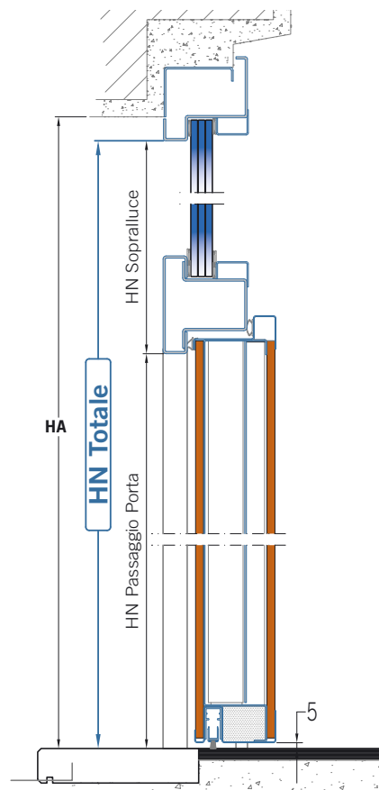
SEZIONE VERTICALE, PORTA CON SOPRALUCE FISSO, SOGLIA TIPO"1" VERTICAL CROSS-SECTION, DOOR WITH FIXED TRANSOM, TYPE "1" THRESHOLD
